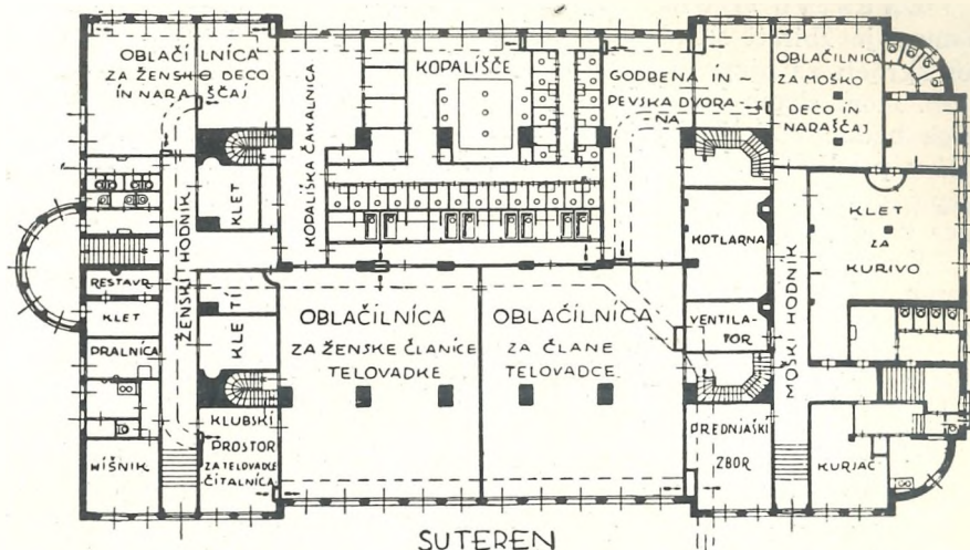
Tloris suterena Sokolskega doma na Taboru
