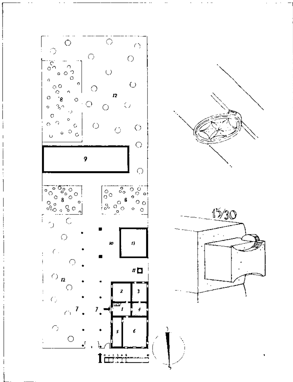
Sl. 1. Situacija in tlnčrt hiše št. 5 »pri Smukoviču« v Pekrah.
