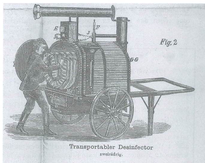
Premični parni razkužilni aparat podjetja W. E. Thursfield z Dunaja, za katerega se je leta 1887 zanimala občina Škofja Loka. (SI_ZAL_ŠKL/0063, Občina Škofja Loka, t. e. 131)
