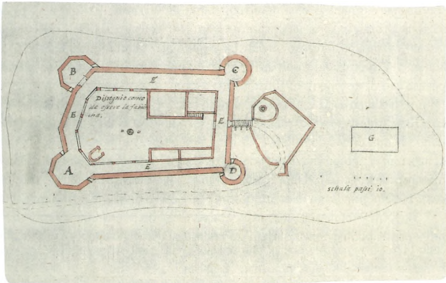
Slika 2. Tloris tolminskega gradu Kozlov rob, "kot mora biti izgradnja" (beneški načrt prenove pred prvo avstrijsko-beneško vojno, najkasneje 1508). ASV, P. Camera Confini, b. 220, dis. 5.
