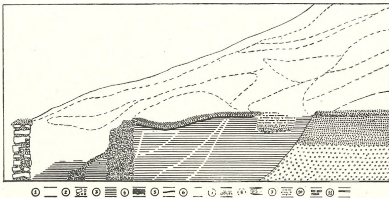
Sl. 5. Profil I—I' ob severni steni rova na zahodnem pobočju Gradu v Ptuj (skica). Orientacija: zahod (levo) — vzhod (desno). Legenda: 1 Erozijski in nasipni sloji. 2 Zid. 3 Antični nasipni sloji. 4 Ožganina. 5 Oglenina. 6 Beli tlak na desnem robu profila takoj na sloju 7. 7 Estrih, 8 Prodniki, pesek. 9 Sip. 10 Antična opeka. 11 Merilo v metrih.
