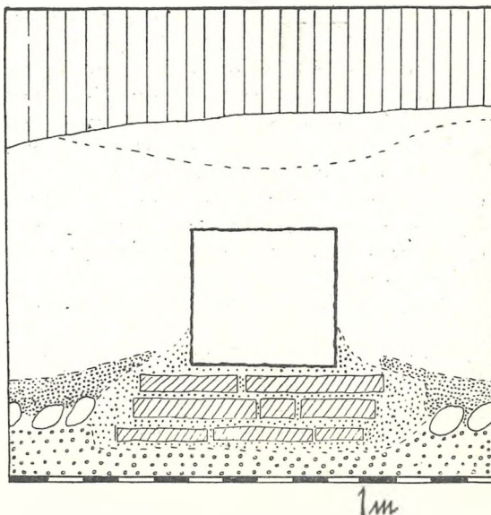
Sl. 4. Blok 1 prezidan z belim tlakom, prim. sl. 5/2 ter legendo na sl. 3.
