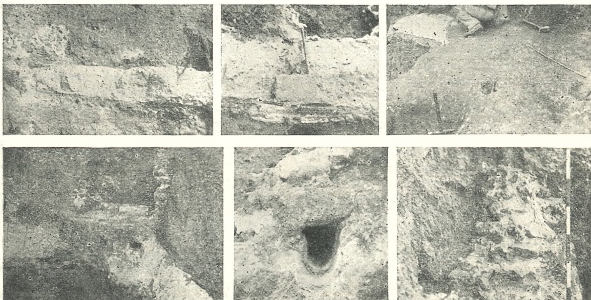
Sl. 5. 1 — Zahodno pobočje Gradu v Ptuj, zaključna stena izkopa vhodnega rova. Na sliki viden prerez 80 cm debelega belega tlaka, pod njim pas rdečega, ki leži na sloju prodnikov. 2 — Blok 1 prežidan z belim tlakom, prim. sl. 4. 3 — Površina belega tlaka; v njej vidni dve manjši jami. 4 — Pogled na rimsko pobočno škarpo z odtočnimi kanali. 5 — Drenažni propust v pobočni škarpi. 6 — Prerež pobočne škarpe.
