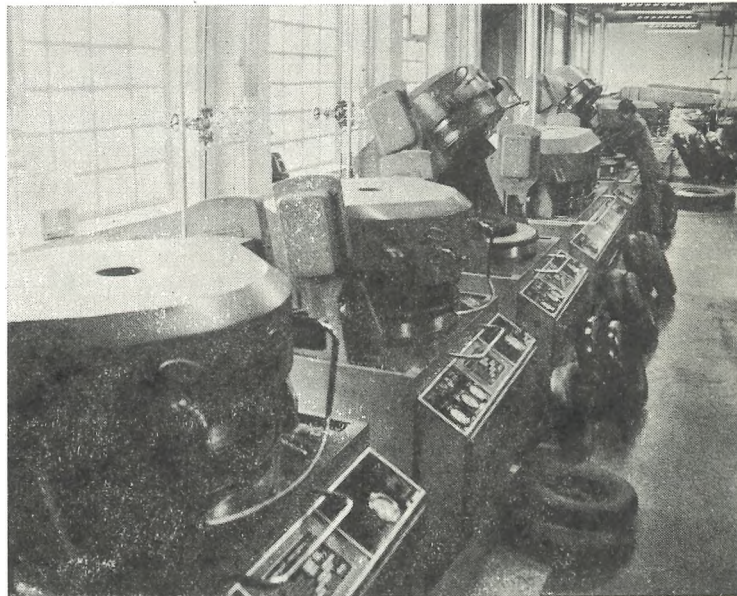
Linija za vulkanizacijo avtomobilskih plaščev
