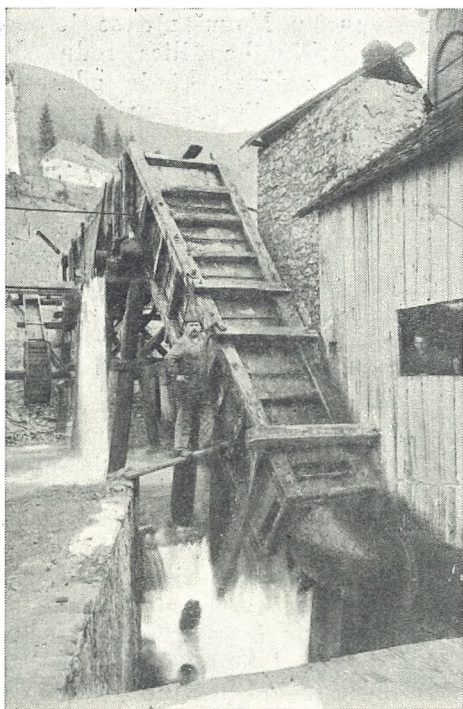
Speljava vodnega pogona valjavnične turbine v Sp. fužini 1876–1908. Ob njem stoji mojster Valentin Solar, v liniji je Janez Lazar. Zidovje stare fužine
