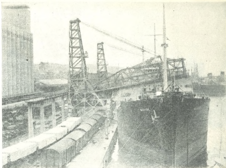
Prekladalni mostovi tranzitnega žitnega silosa na Reki, ki jih je zgradila »Metalna« v Mariboru, s kapaciteto 400 t/h, sodijo med največje v Evropi
